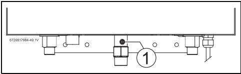
Fig. 36 Port d'essai de pression du gaz
