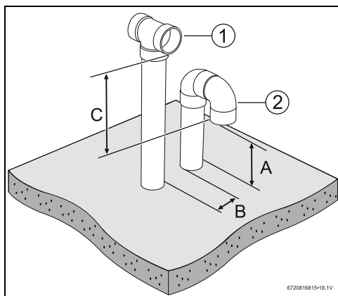
Fig. 13 Système de ventilation verticale
