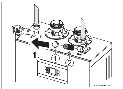
Fig. 29 Filtre à eau
