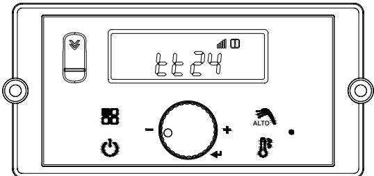
2. Seleccione tt24 u OndE
