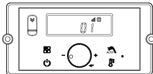
4. Seleccione el tiempo de funcionamiento (de 01 a 60 minutos)** **Esto establecerá cuánto tiempo funcionará la bomba del climatizador en cada ciclo antibacterias.
