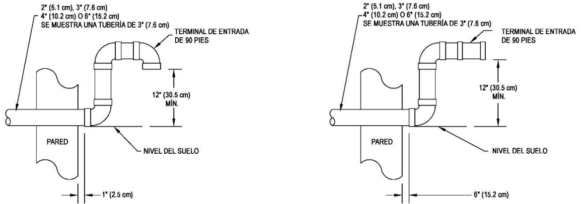
Figura 17: Terminal de la ventilación (poca distancia al suelo)
