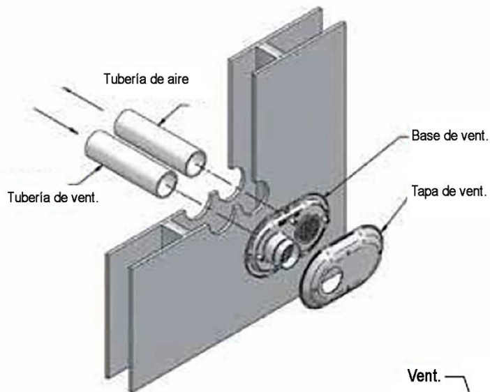
Figura 26: Montaje de la terminación en pared lateral
