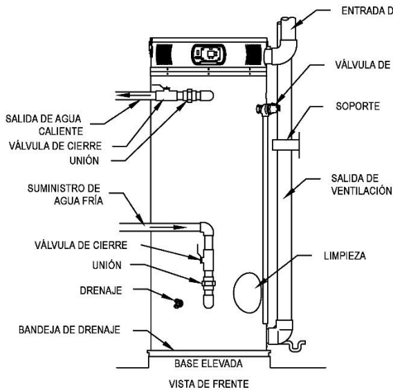
Figura 4: Conexión típica de la entrada frontal
