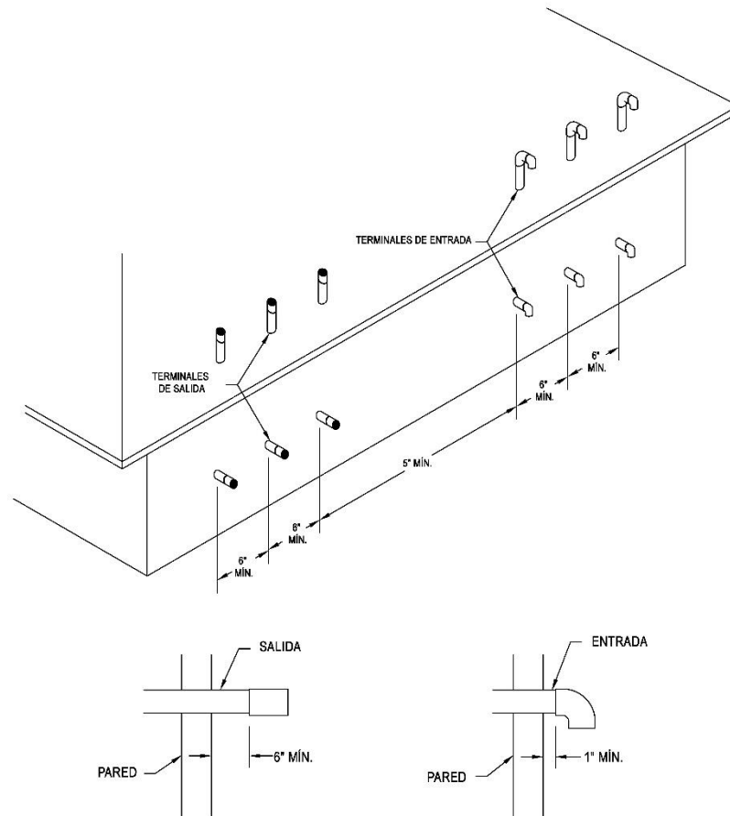
Figura 17: Terminal de la ventilación (poca distancia al suelo)
