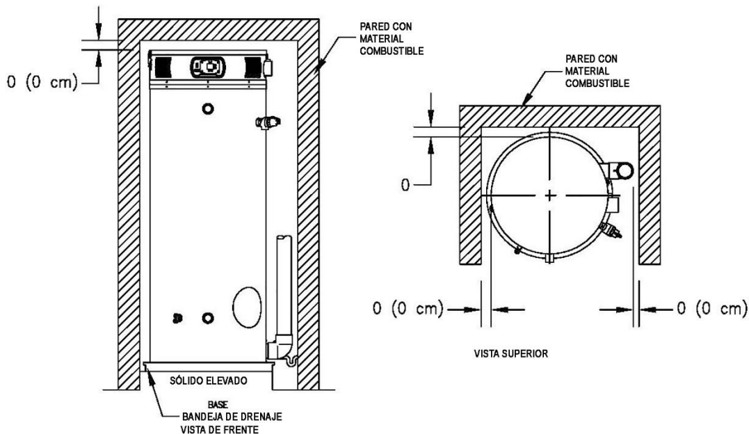
Figura 3a: Distancias mínimas al material combustible
