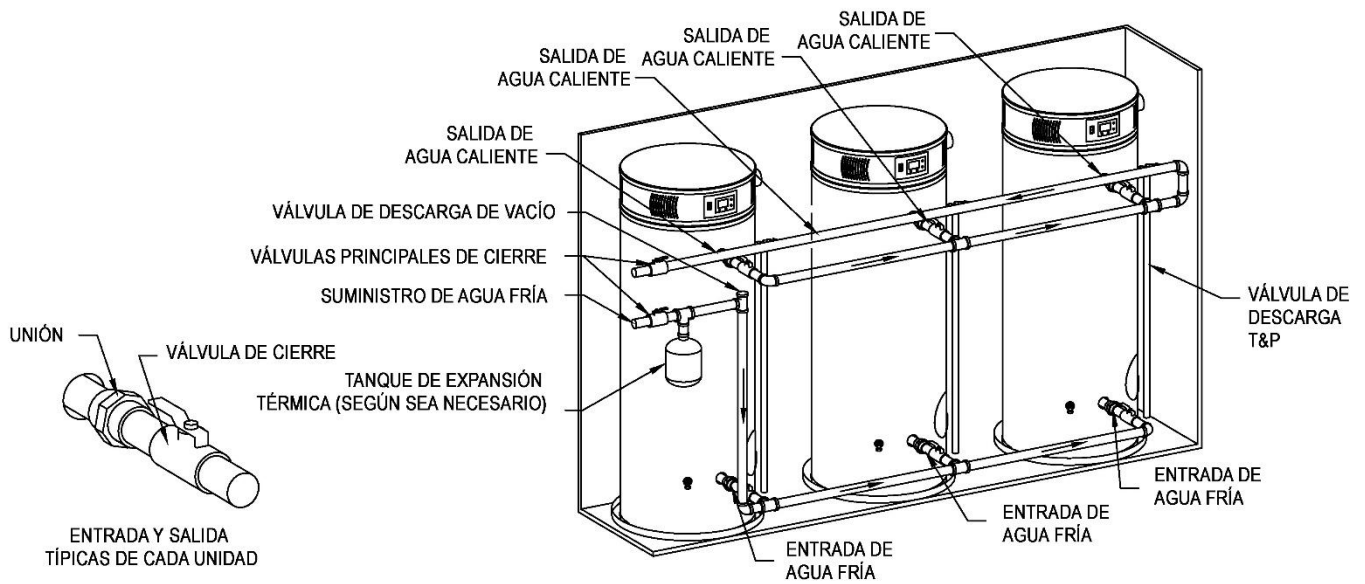
Figura 7: Conexión típica de tres calentadores de agua
