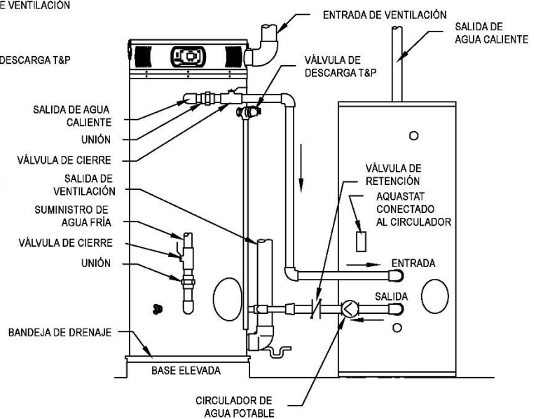
Figura 5: Conexión típica de la entrada frontal con calentador de almacenamiento
