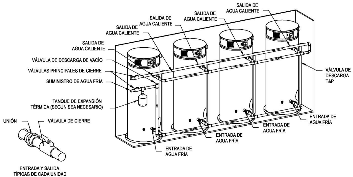
Figura 8: Conexión típica de cuatro calentadores de agua
