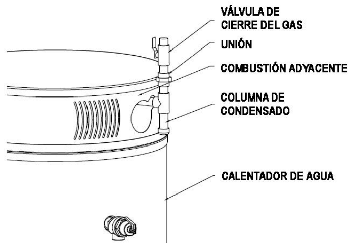
Figura 28: Columna de condensado
