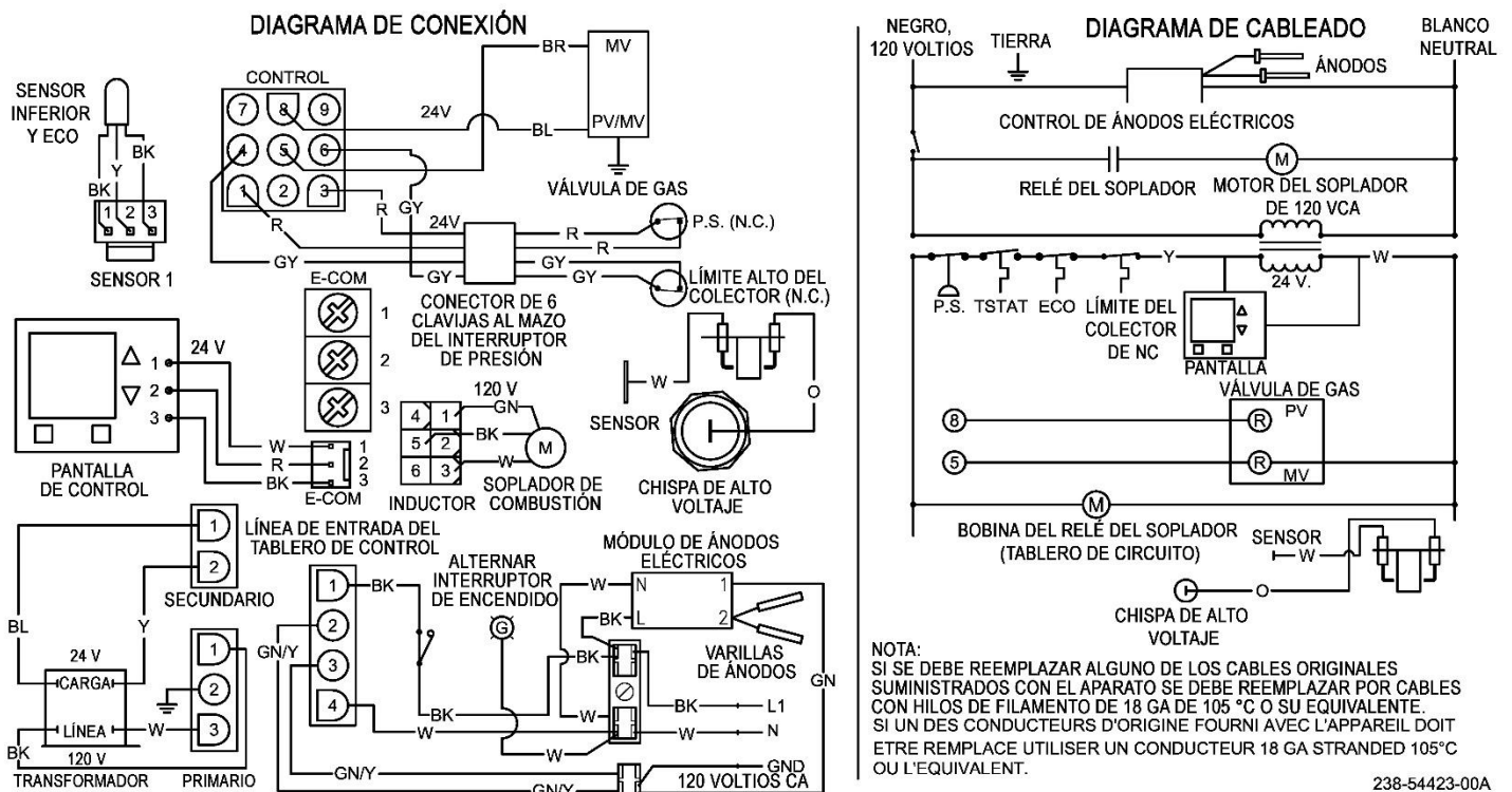
Figura 29: Diagrama de cableado y esquema
