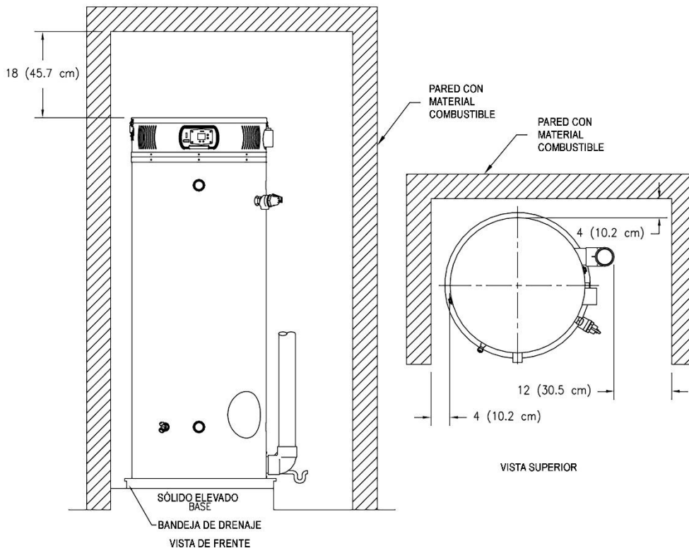
Figura 3b: Distancias mínimas recomendadas para el acceso para las reparaciones
