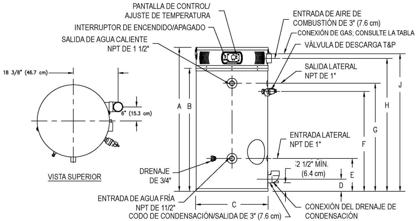
Figura 1: Disposición dimensional
