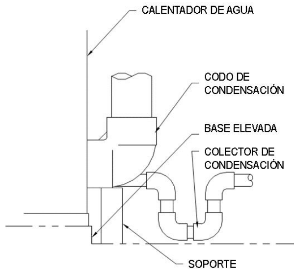
Figura 2: Codo de condensación con colector
