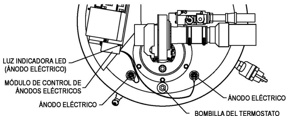
Figura 32: Ubicaciones de los ánodos eléctricos
