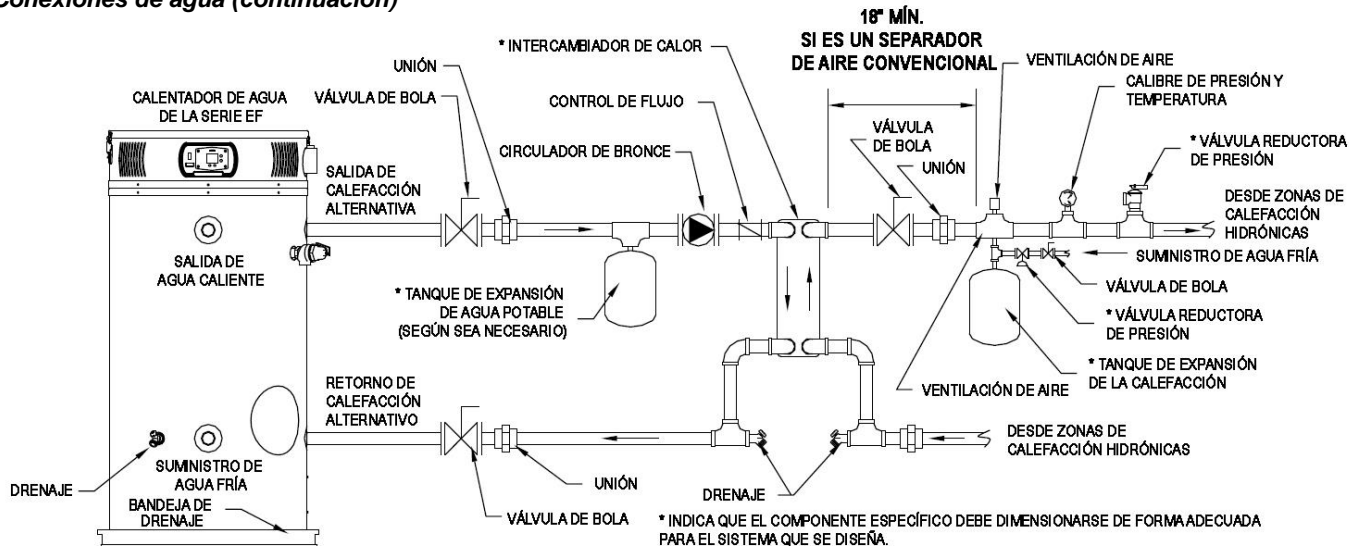
Figura 10: Esquema típico de plomería para calefacción por zonas
