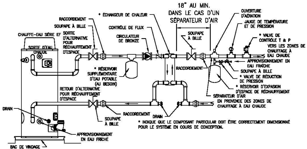
Figure 10 — Schéma type de plomberie pour le chauffage par zone
