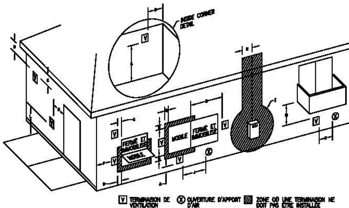
Figure 11b — Dégagements des bornes de ventilation directe et de ventilation directe motorisée (évent direct, entrée et sortie)
